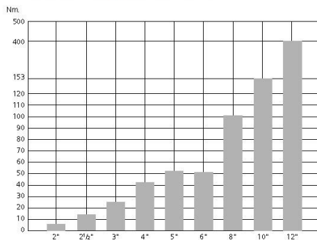
Вафельные дроссельные клапаны с седлом из EPDM
