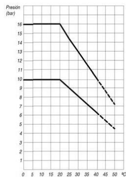
Диаграмма давление-температура для фитингов PEHD
