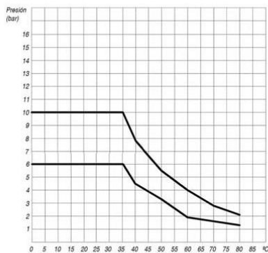
Диаграмма давление-температура для фитингов из полипропилена
